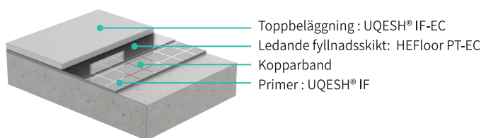
Schematisk uppbyggnad
