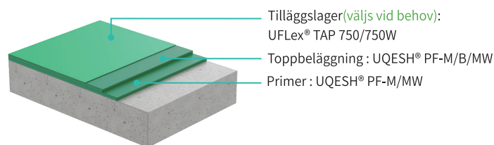
Schematisk uppbyggnad
